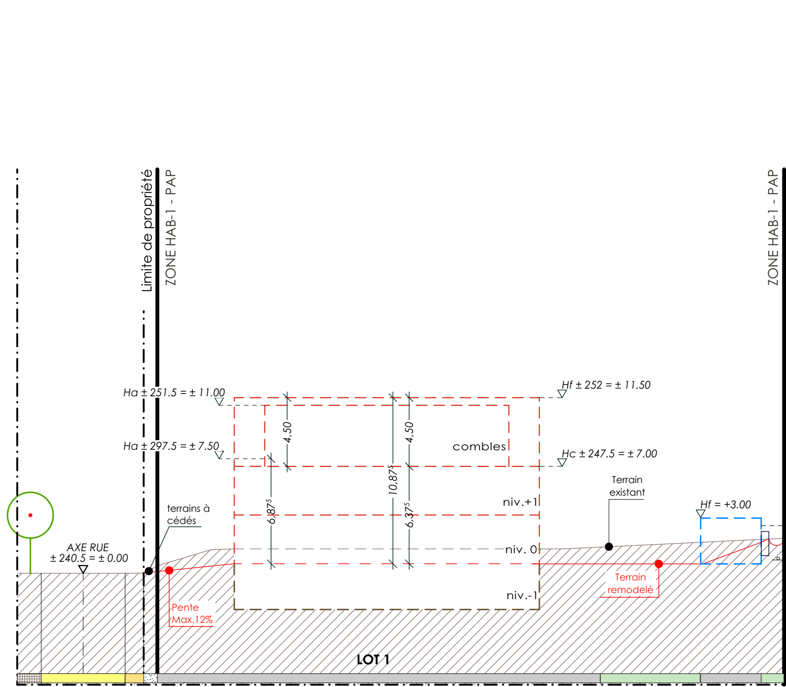
COUPE SIGNIFICATIVE TRANSVERSALE BB'
