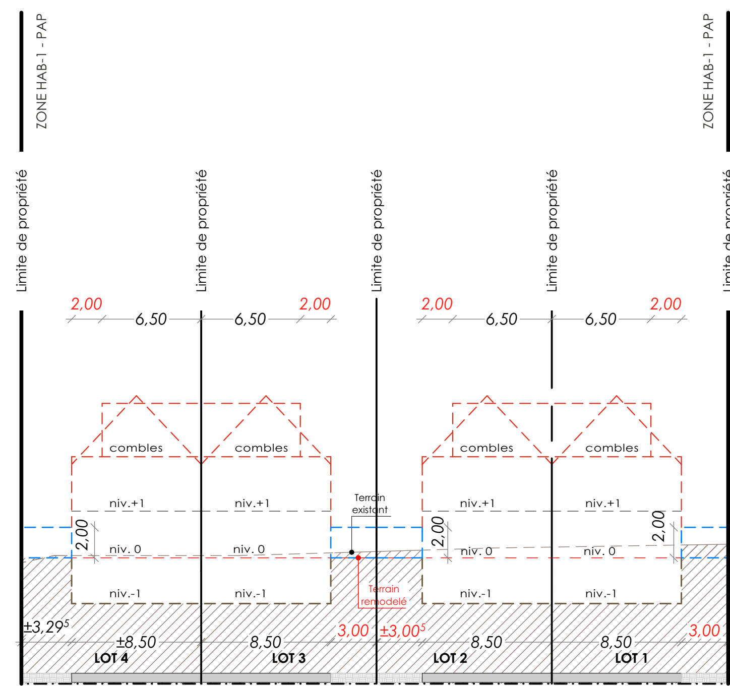
COUPE SIGNIFICATIVE LONGITUDINALE AA'
