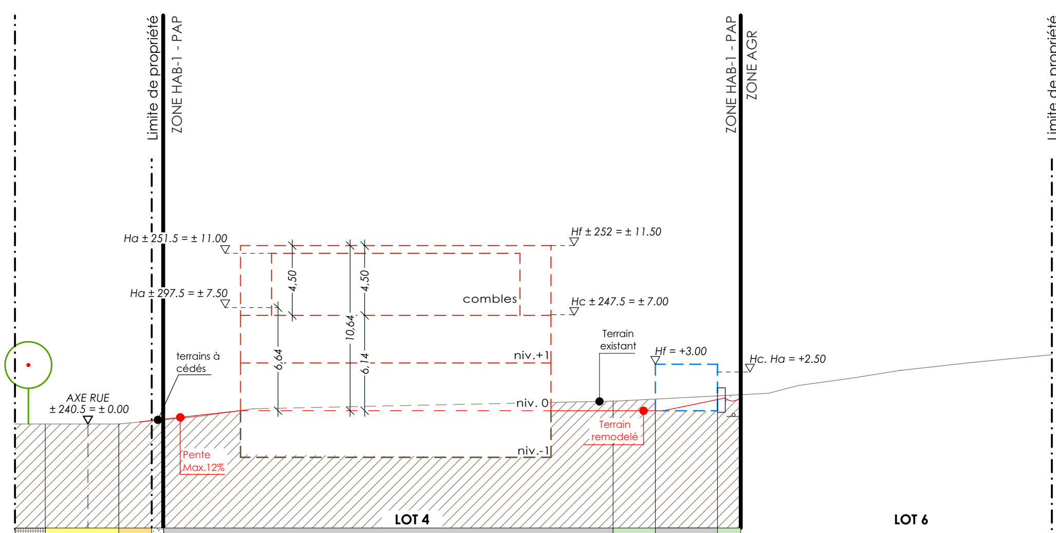
COUPE SIGNIFICATIVE TRANSVERSALE EE'
