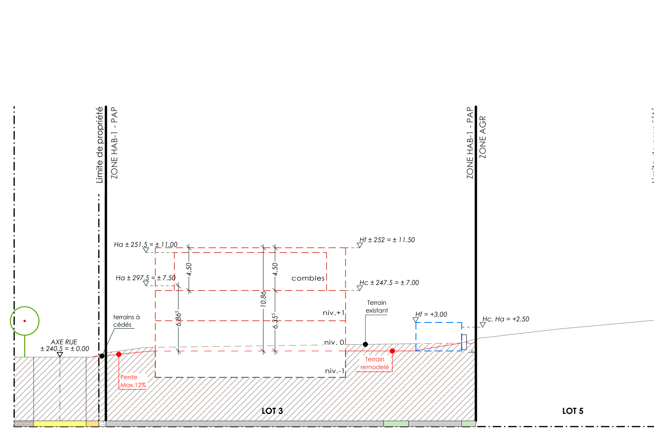
COUPE SIGNIFICATIVE TRANSVERSALE DD'
